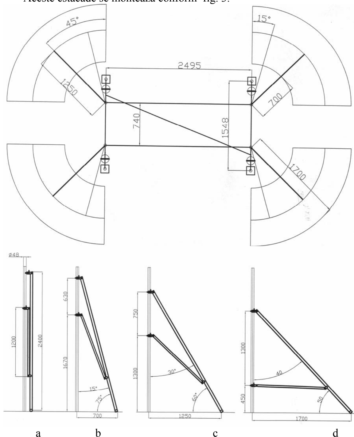
Fig. 3 – Montarea estacadelor
