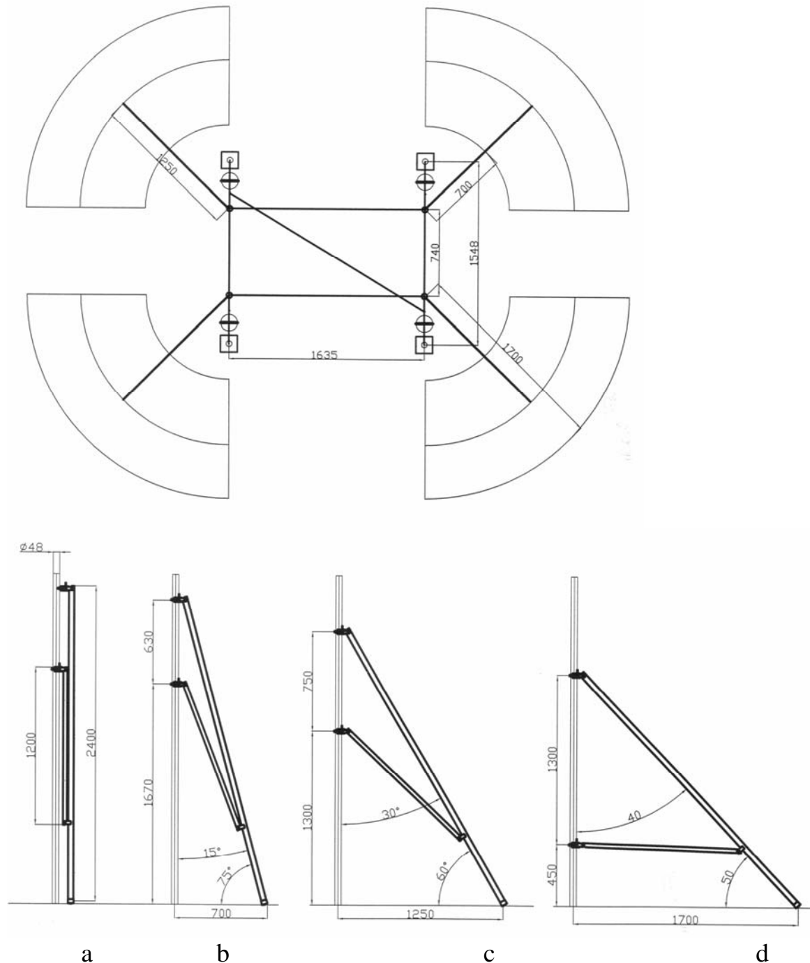
Fig. 3 – Montarea estacadelor
