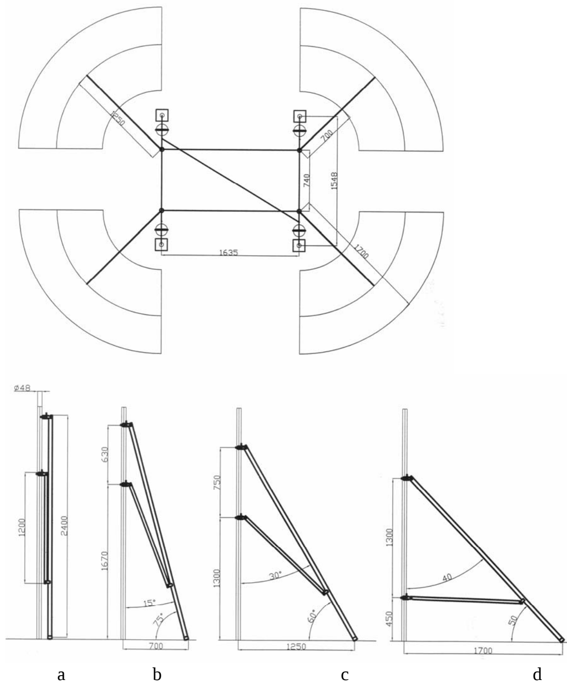
Fig. 3 – Montarea estacadelor
