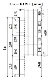
SCARA PISICA RARIS, ASAMBLABILA, INOX cod SP5A
