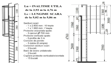
SCARA PISICA RARIS. ASAMBLABILA, ALUMINIU, tip SP1AA
